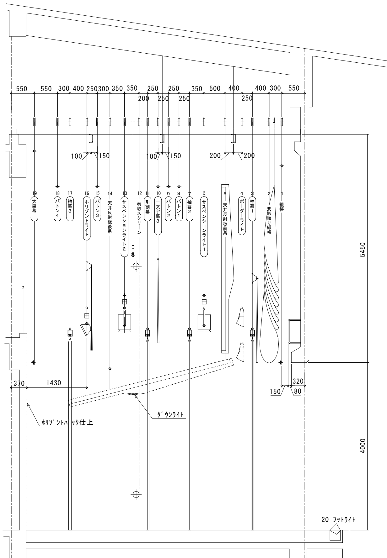
能代市文化会館中ホール 吊物断面図
